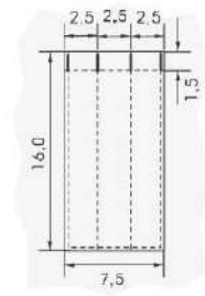
Figura 13 - Detalhes da bolsa auxiliar tipo caneteiro
