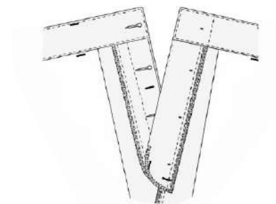
Figura 12 - Detalhes internos da braguiha
