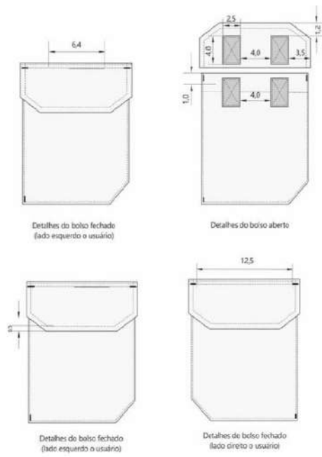
Figura 7 – Detalhes dos bolsos camisa tática
