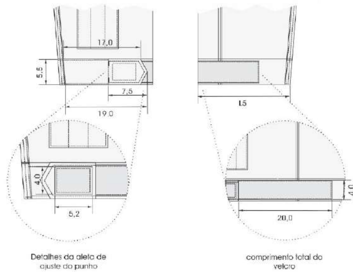
Figura 14 - Detalhes do punho
