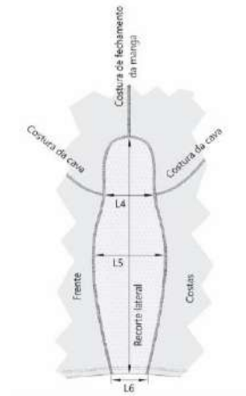
Figura 10 – Detalhes do recorte lateral da camisa tática
