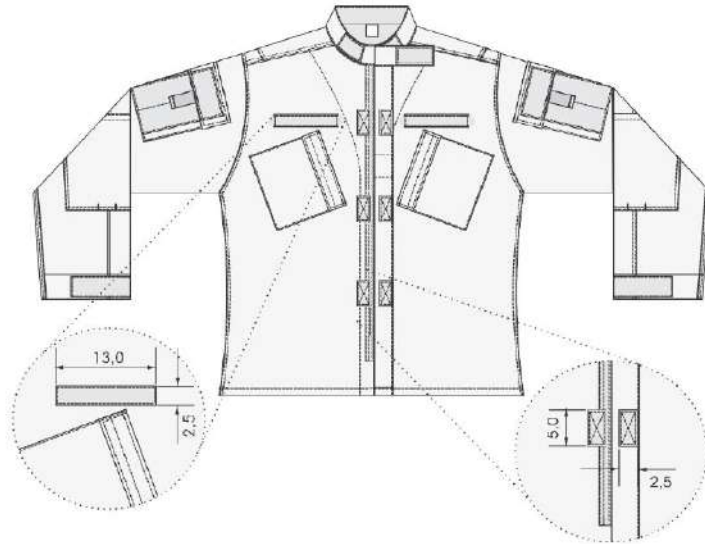
Figura 5 - Detalhes dos veloros e da abertura frontal
