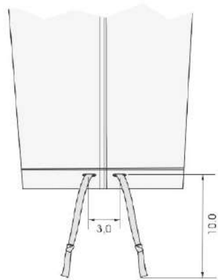
Figura 20 - Detalhes internos da bainha
