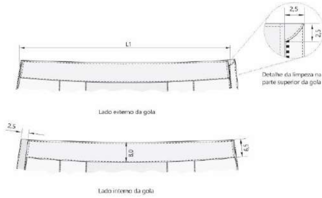
Figura 5 – Detalhes da gola camisa tática
