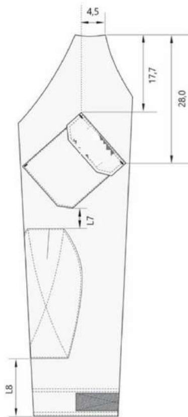
Figura 12 – Detalhes dos bolsos e reforço cotovelo das mangas
