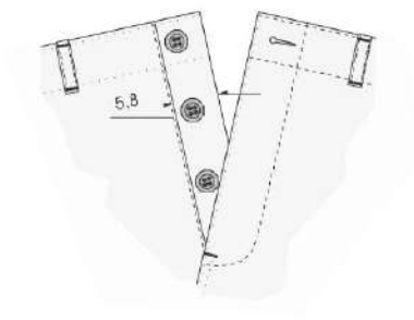
Figura 11 - Detalhes da braguiha aberta
