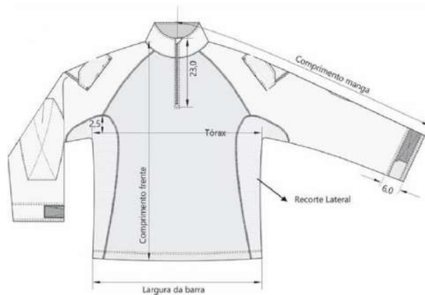
Figura 1 – Detalhes da camisa tática
