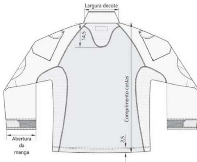
Figura 3 – Detalhes da camisa tática Medidas em cm
