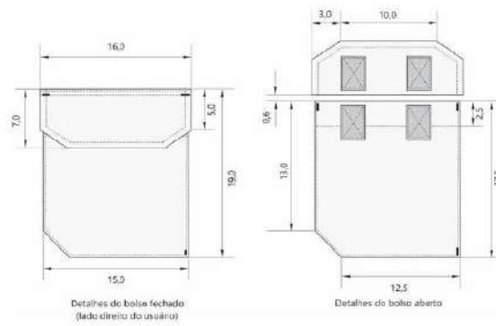
Figura 8 – Detalhes dos fechos de contatos (velcro) dos bolsos camisa tática Medidas em cm
