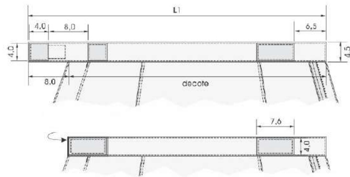
Figura 4 - Detalhes da goia
