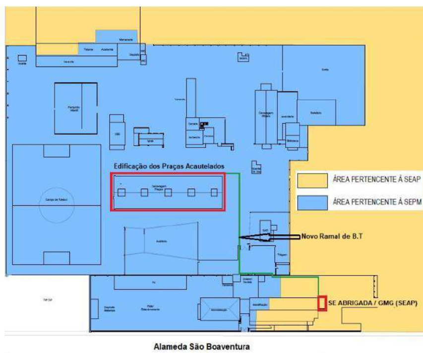
Figura 01 - Edificação contemplada com as benfeitorias elétricas, o posicionamento do novo ramal de B.T a ser projetado e instalado, a SE Abrigada e o GMG.
