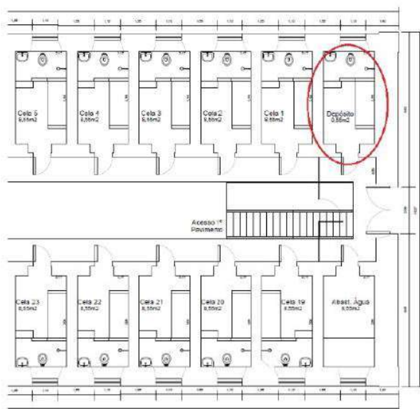
Figura 03 – Detalhe marcado em linhas de contornos na cor vermelha, no espaço onde deverá ser instalados os novos Quadros de Distribuição para atender a edificação.
